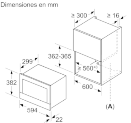
A: Pared trasera abierta
