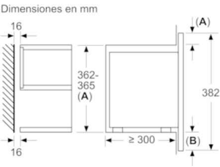
A: Saliente superior: Hueco 362: 6 mm Hueco 365: 3 mm B: Saliente inferior: 14 mm
